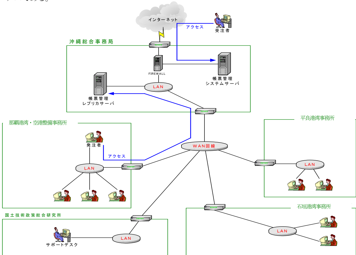
システム利用におけるネットワーク構成図
