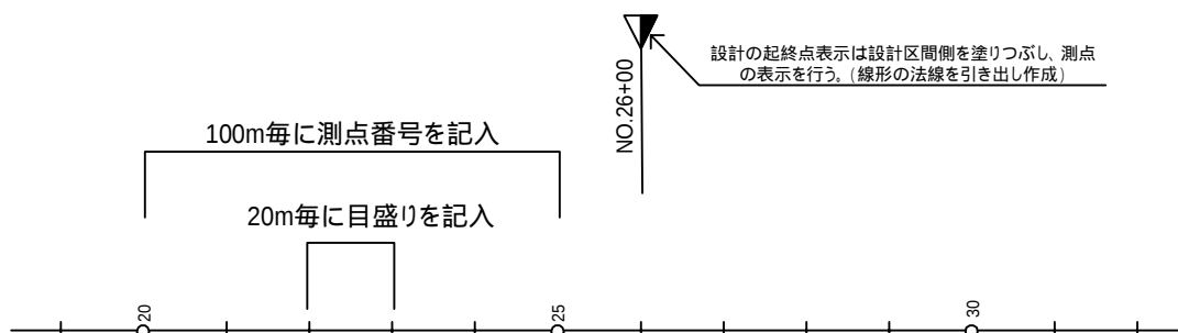
図 2-1 平面線形の表現方法
