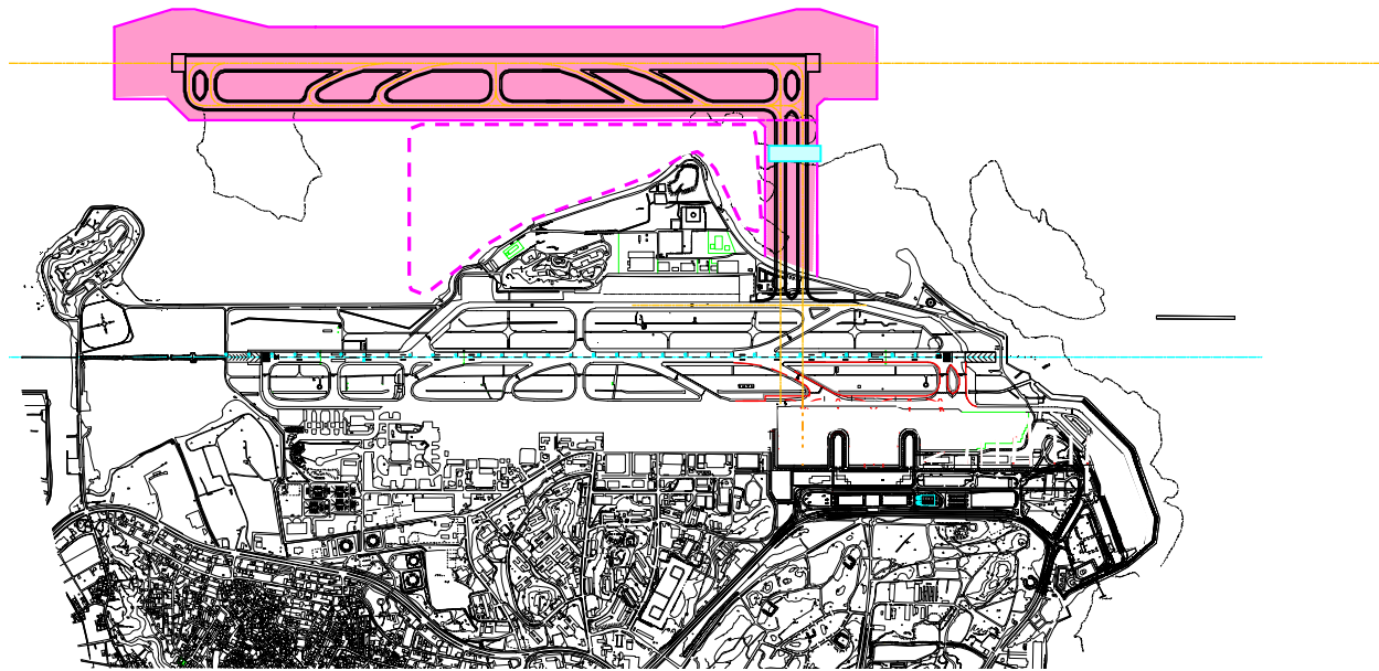
滑走路間隔1310m
