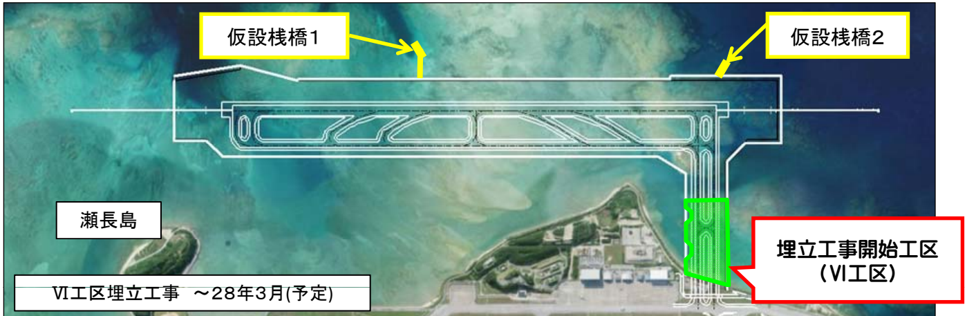
VI工区護岸締切状況(上空から)
