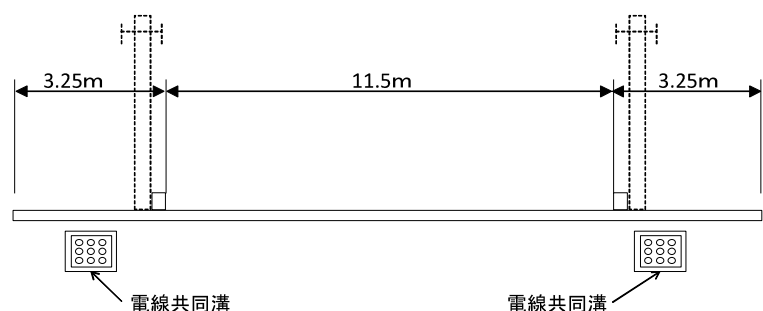
【標準断面図】
