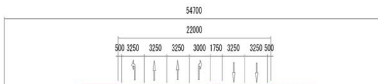
【平面図】
