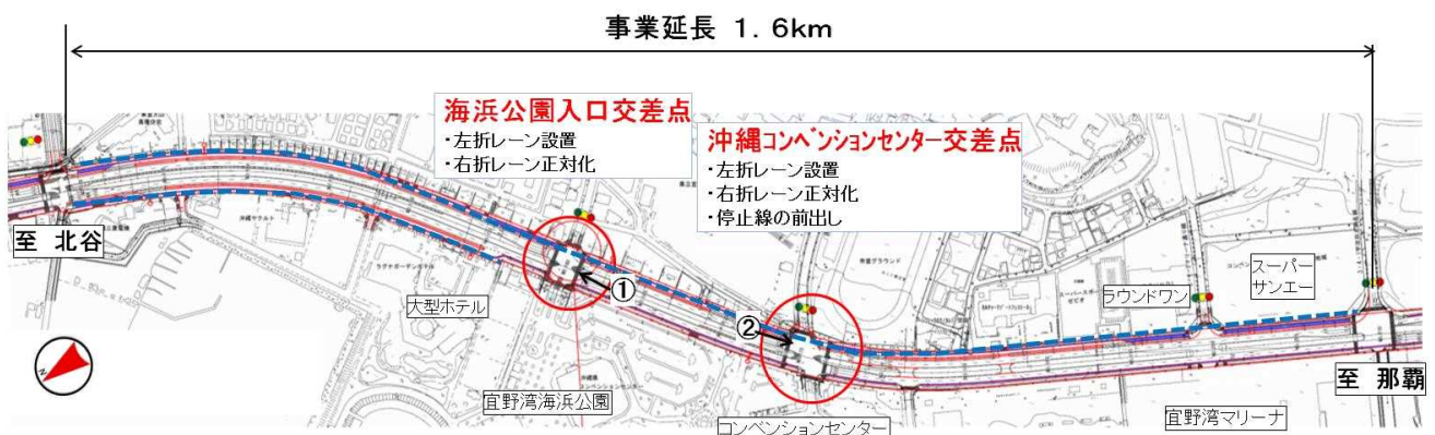
【平面図】
