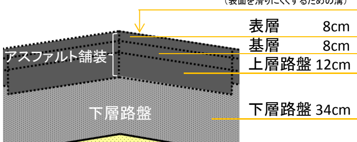
滑走路舗装の標準断面
