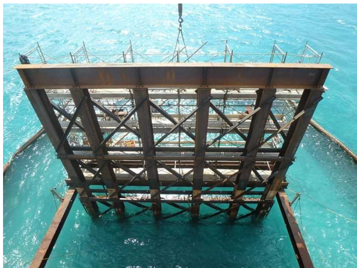
① 【南側進入灯】仮設構台設定状況(平成30年10月撮影)
