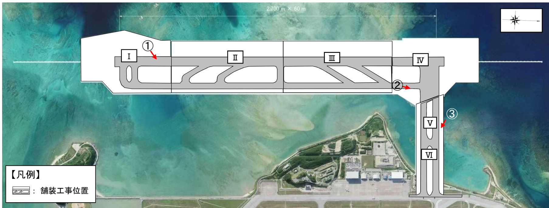
舗装工事の実施位置図
