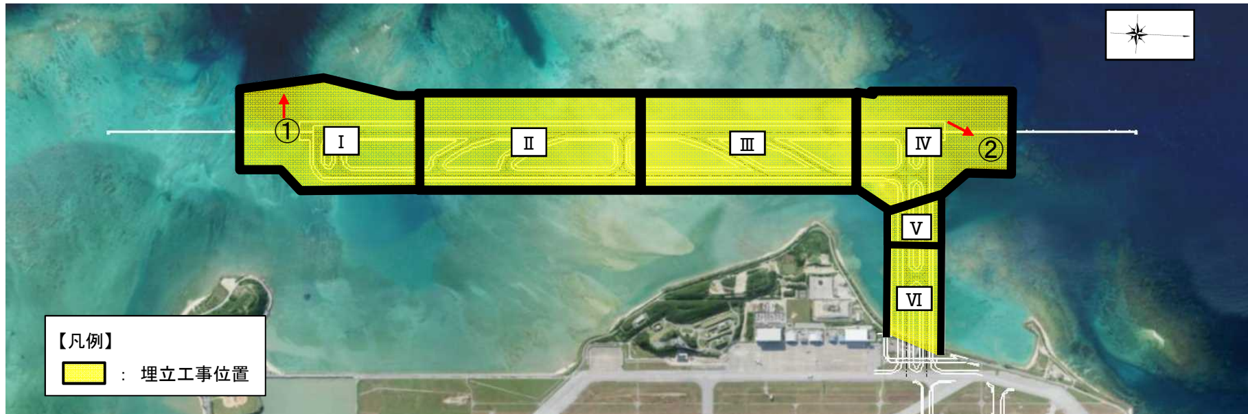
埋立工事の実施位置図
