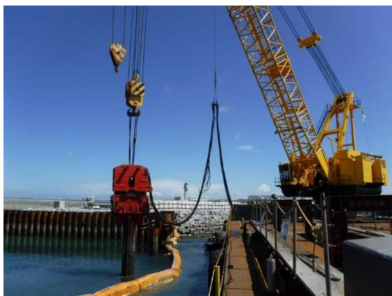
① 【仮設棧橋1撤去】鋼管矢板引抜状況 (令和元年9月撮影)
