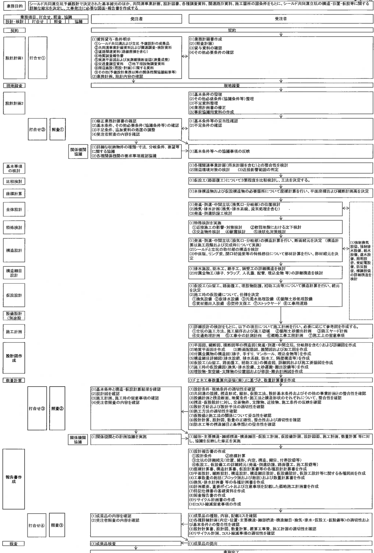
シールド共同溝立坑詳細設計フロー(案)
