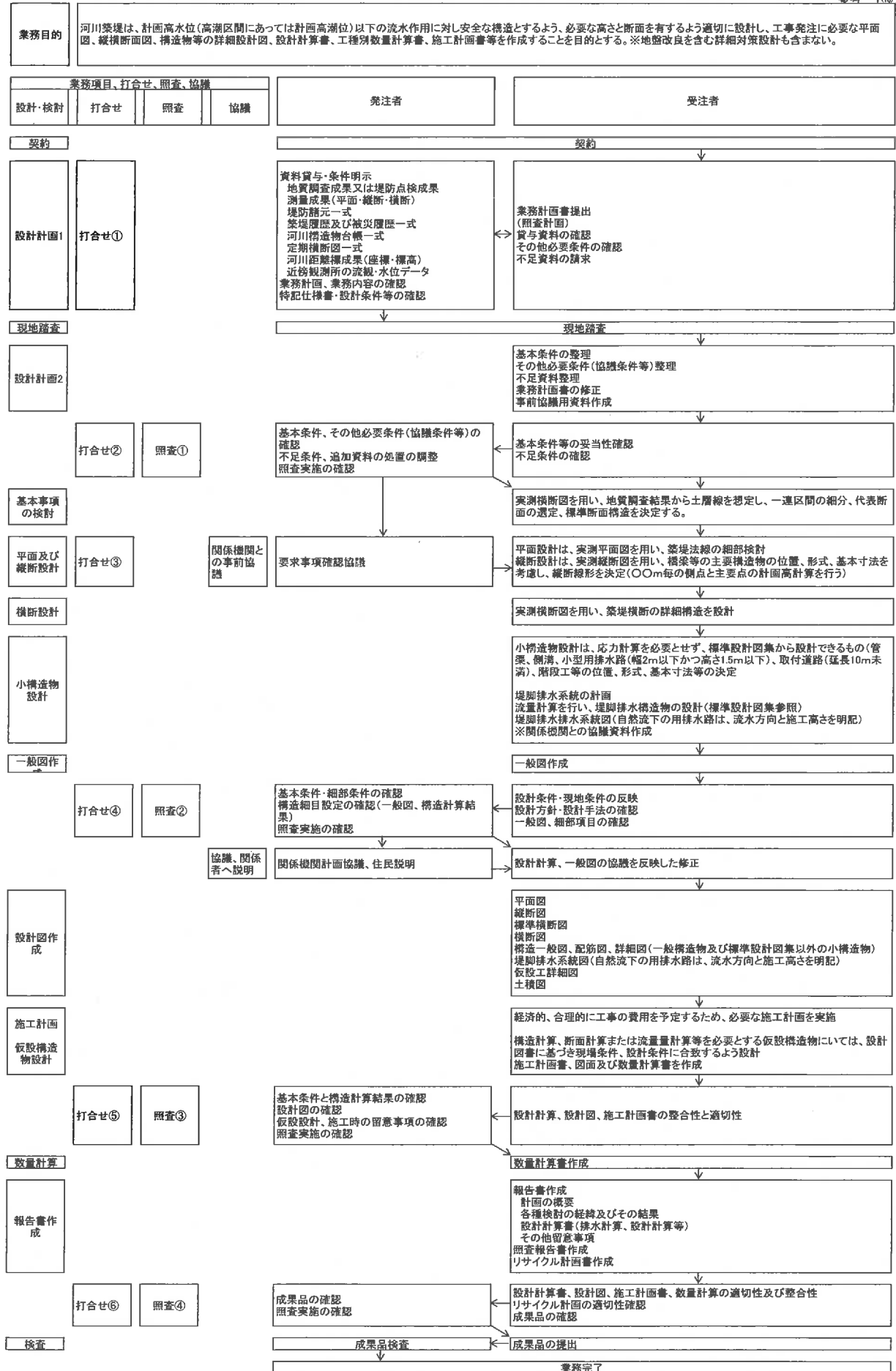
築堤詳細設計フロー(案)
