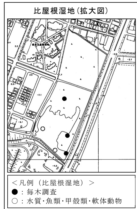
図 2.1.1 環境監視調査 (工事中) の位置図
