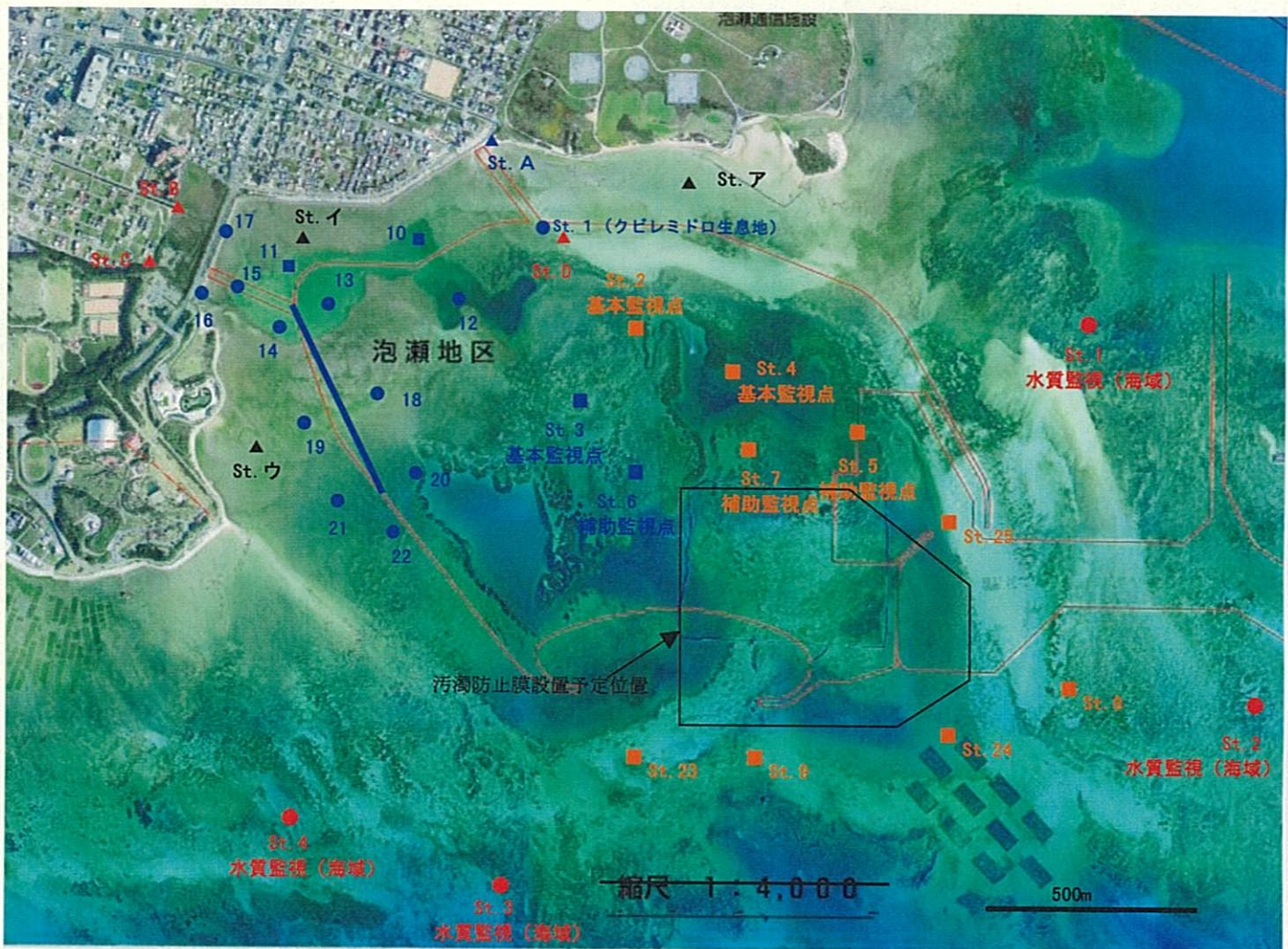
図3 仮設橋梁工事および海上工事の濁り監視地点
