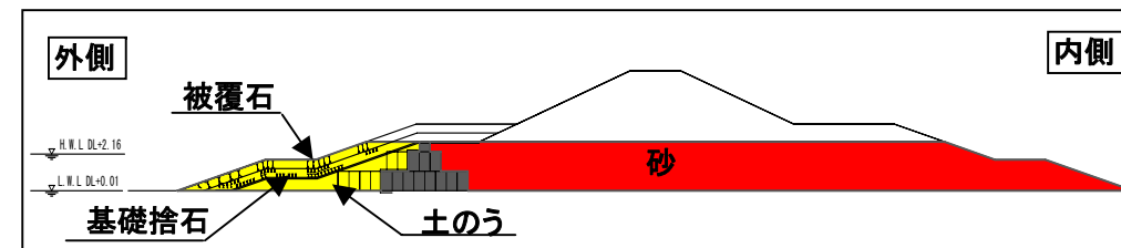
①-①断面図
