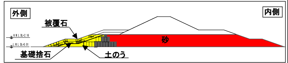
①-①断面図
