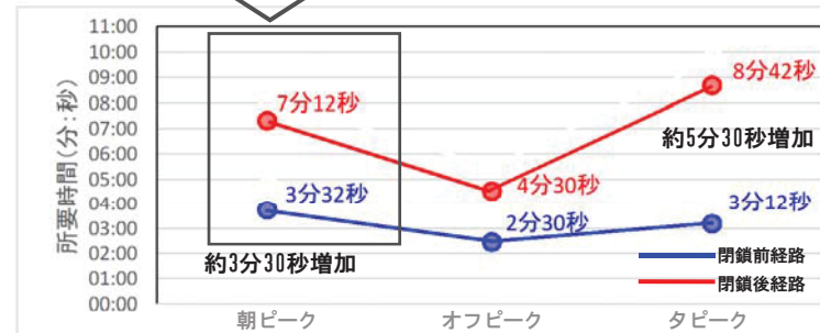
図-11 所要時間 (北側生活エリアから真玉橋交差点)
