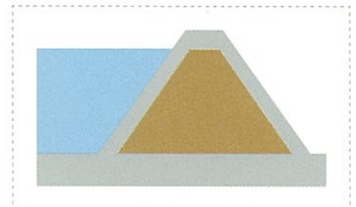
[CSGダム]
