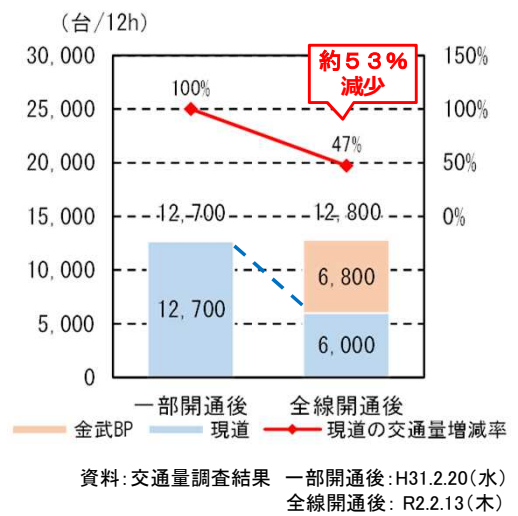
(図1) 交通量の変化 ((仮)金武(北)交差点付近: A-A'断面)
