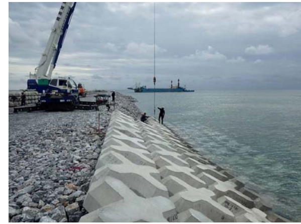
【I工区】被覆ブロック据付状況
