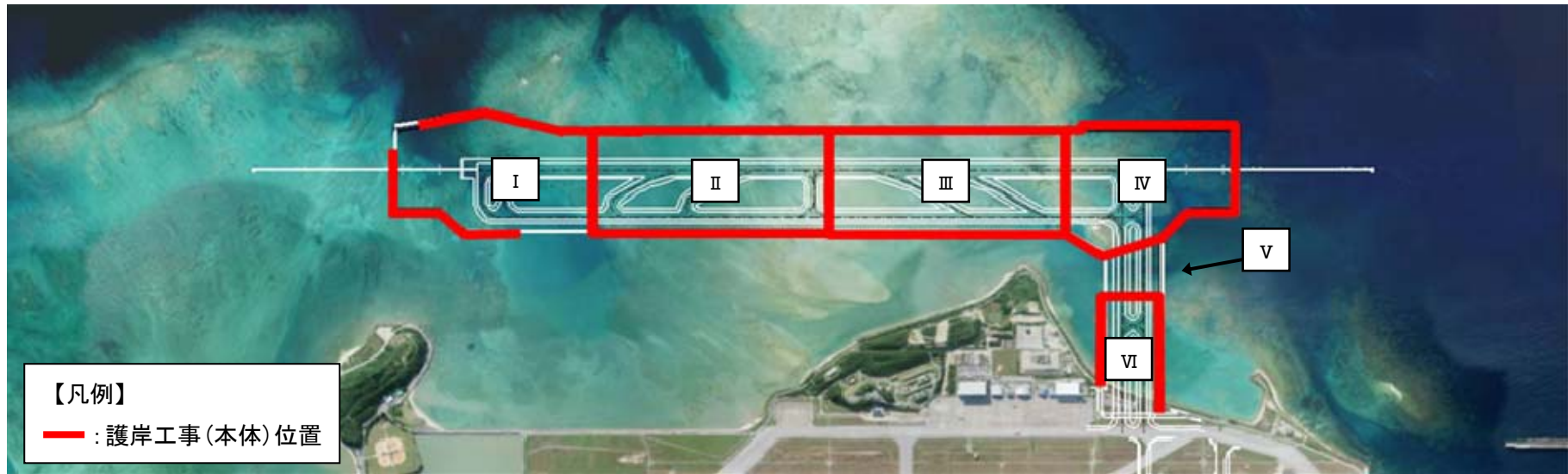
図 4 護岸工事の実施位置
