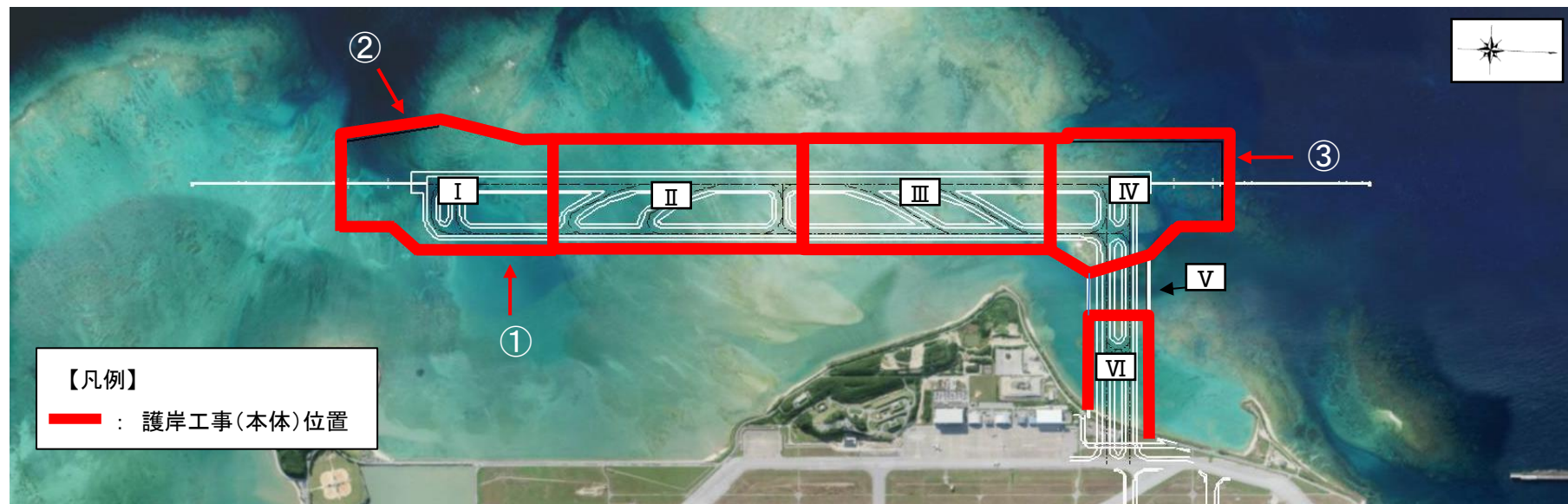
護岸工事の実施位置図
