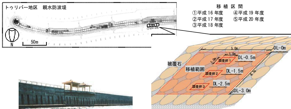
図－4 移植先詳細図
