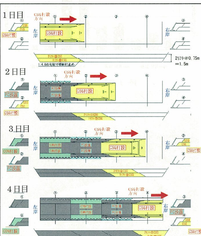
図-8 上位標高部での施工サイクル
