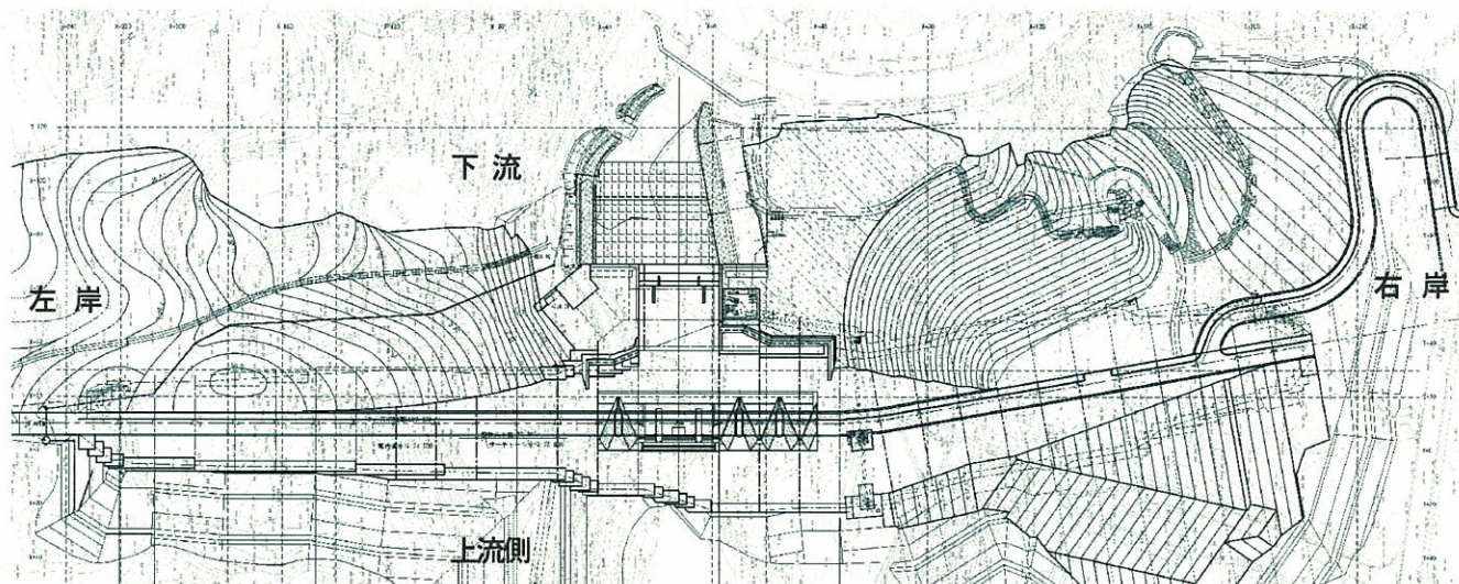
図-3 平面図
