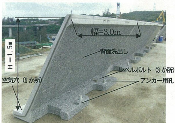
写真-14 PC型枠
