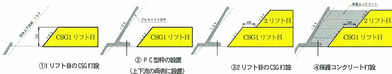
図-6 上下流P C型枠周りでのCSG施工手順
