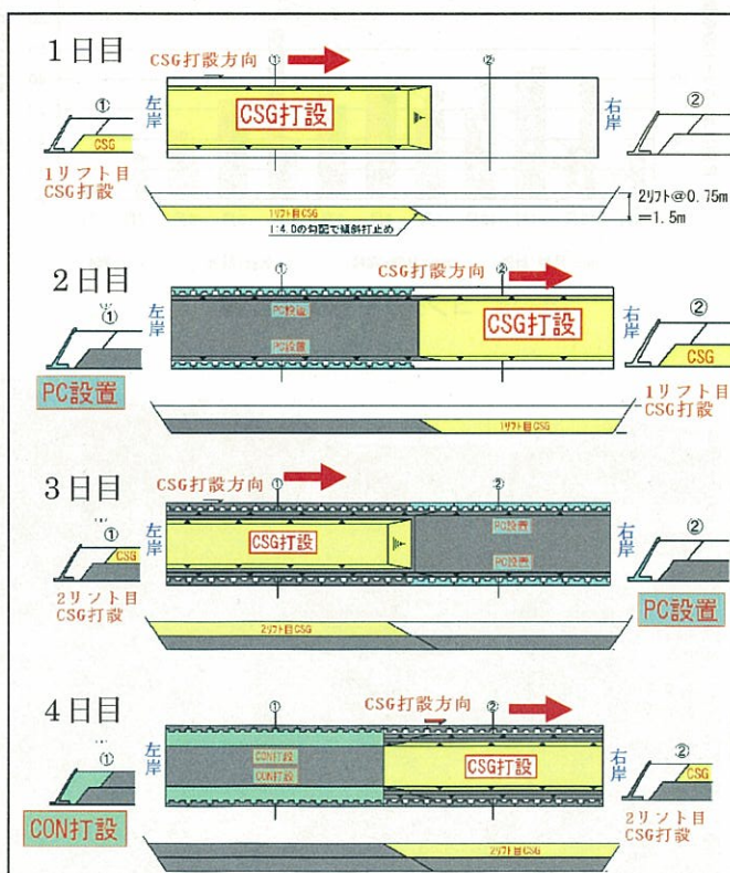
図-7 下位標高部での施工サイクル
