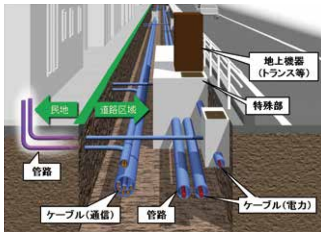
電線共同溝のイメージ
