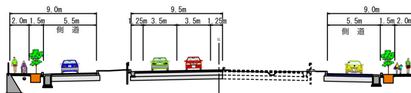
本線平面構造+歩道+側道(県道12号線～親志波平線)
