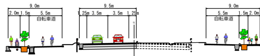
本線平面構造+歩道+自転車道(親志波平線～中央残波線)
