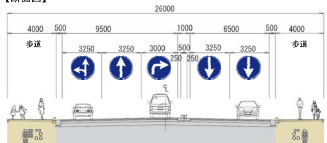
【断面図】
