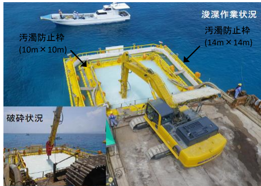
バックホウ浚渫状況
