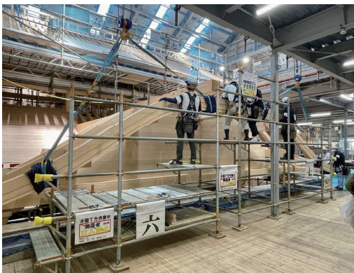
唐破風(正殿2階正面)取付作業の様子(令和6年5月)
