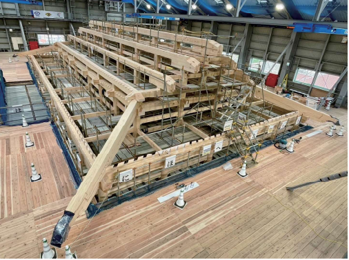
正殿工事 軸組建方完成(令和5年12月)
