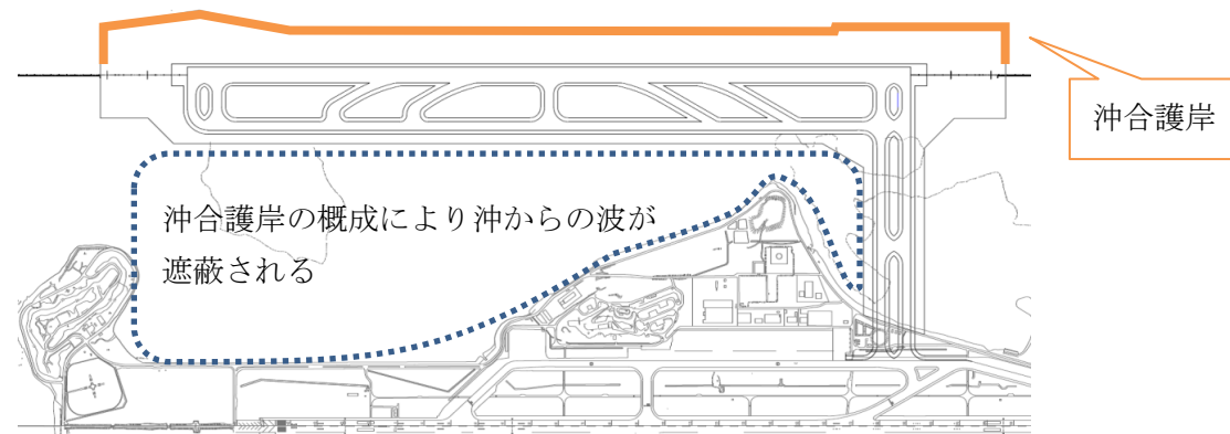
図 16 沖合護岸の位置
