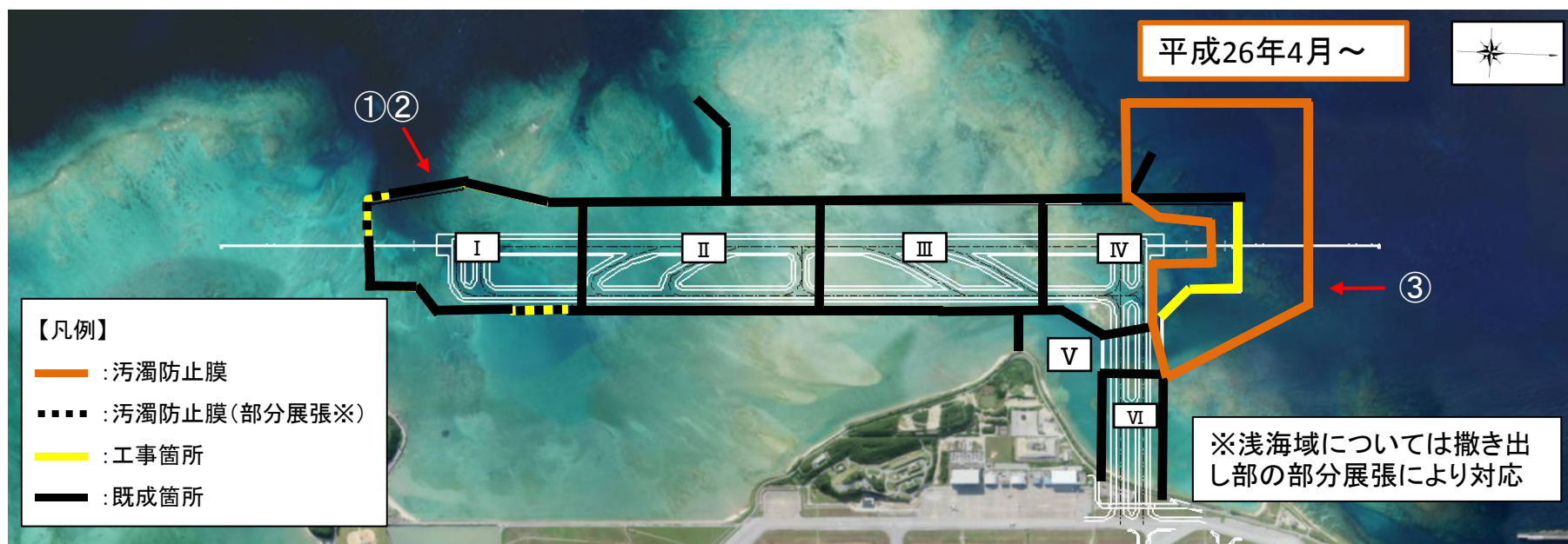
図2 汚濁防止膜の設置位置
