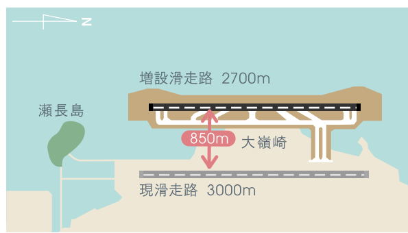
増設 B 案(滑走路間隔850m)
