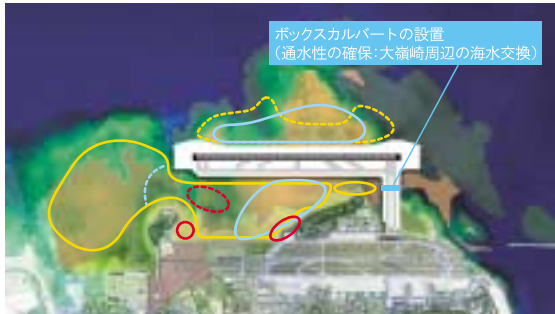
増設A案(滑走路間隔1310m)
