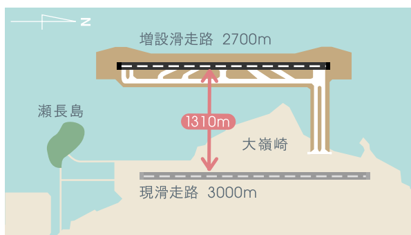
増設 A 案(滑走路間隔1310m)
