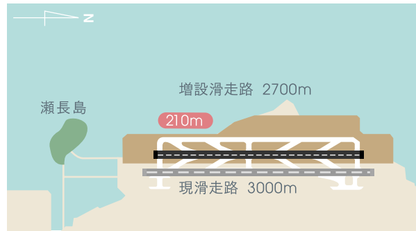
参考(滑走路間隔210m案)
