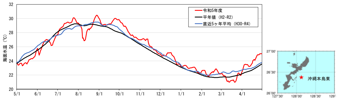
図 2.6.12 沖縄本島東海域における令和5年度海面水温と平年値との比較
