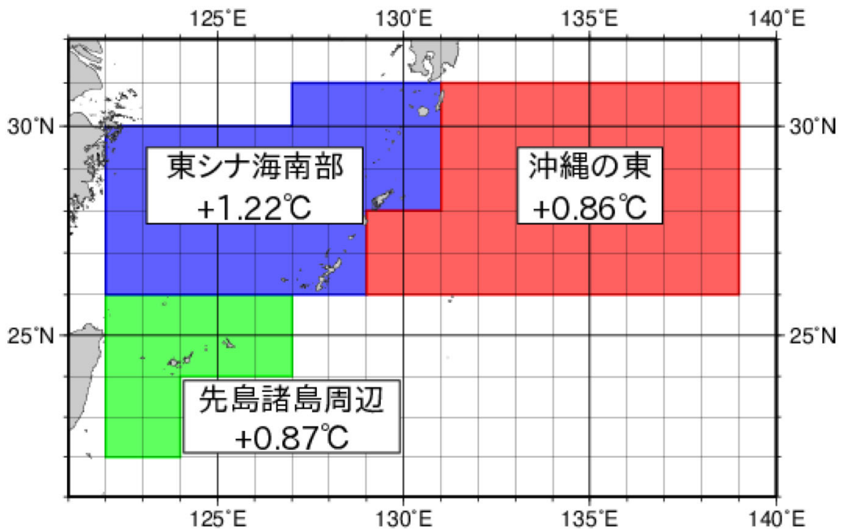
図 2.6.15 沖縄周辺の海域における海域区分と100年あたりの海面水温上昇率
