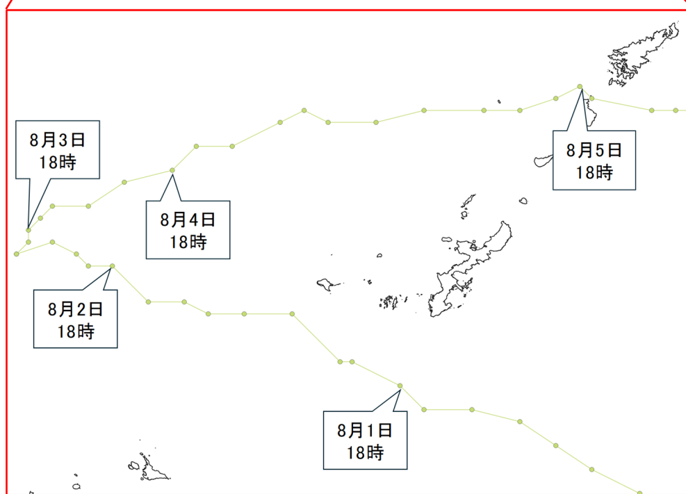
図 2.6.13 台風 6 号の経路
