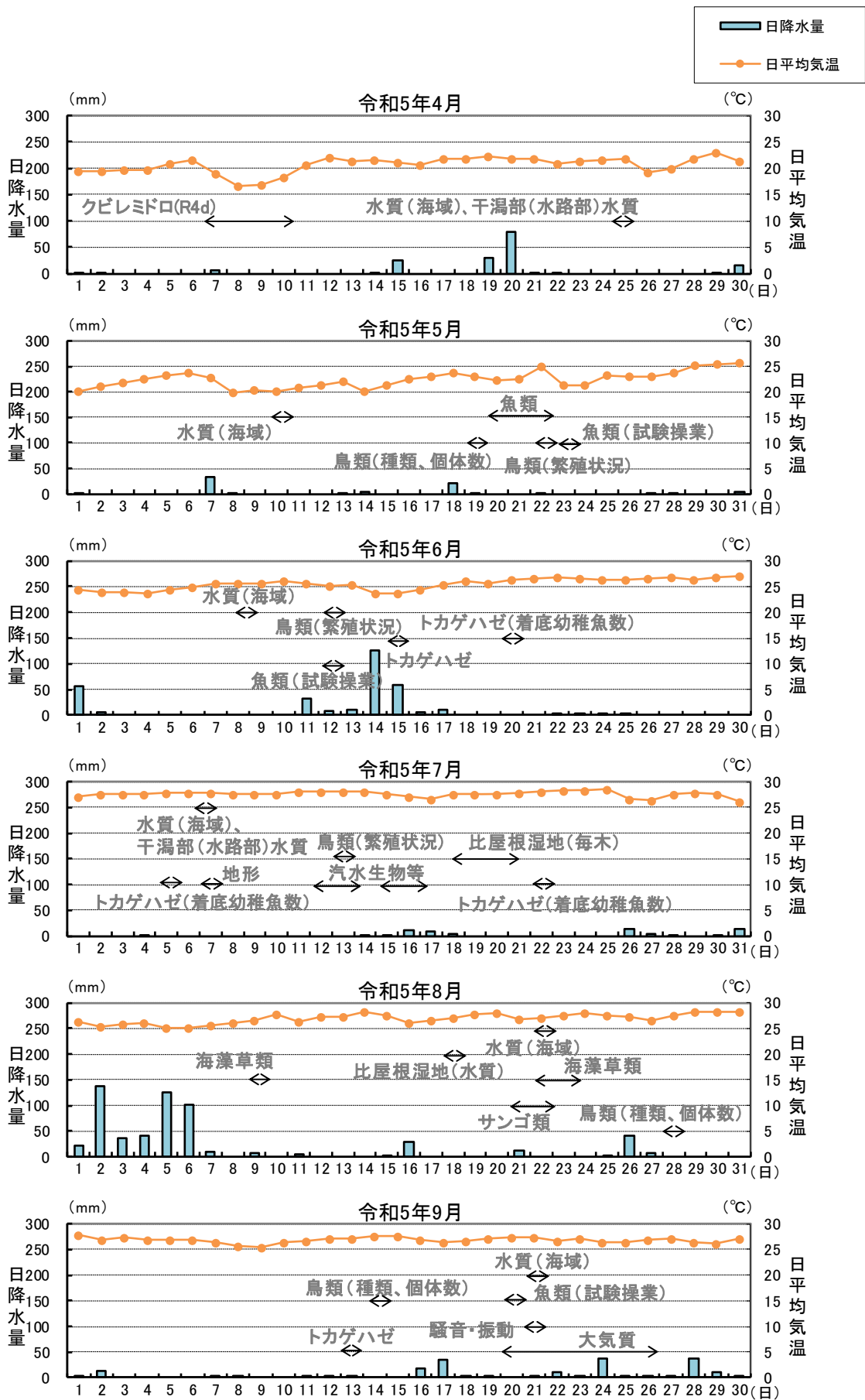
図 1.3.2(1) 調査期間中の日降水量及び日平均気温（令和5年4月～令和5年9月）
