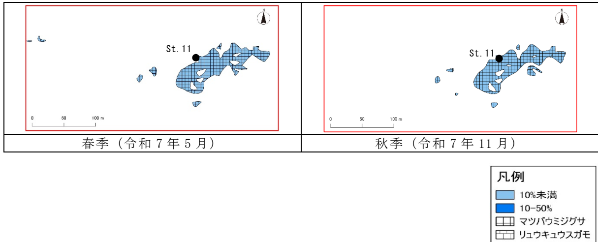
図 2.5.13 小型海草藻場の分布状況の比較
