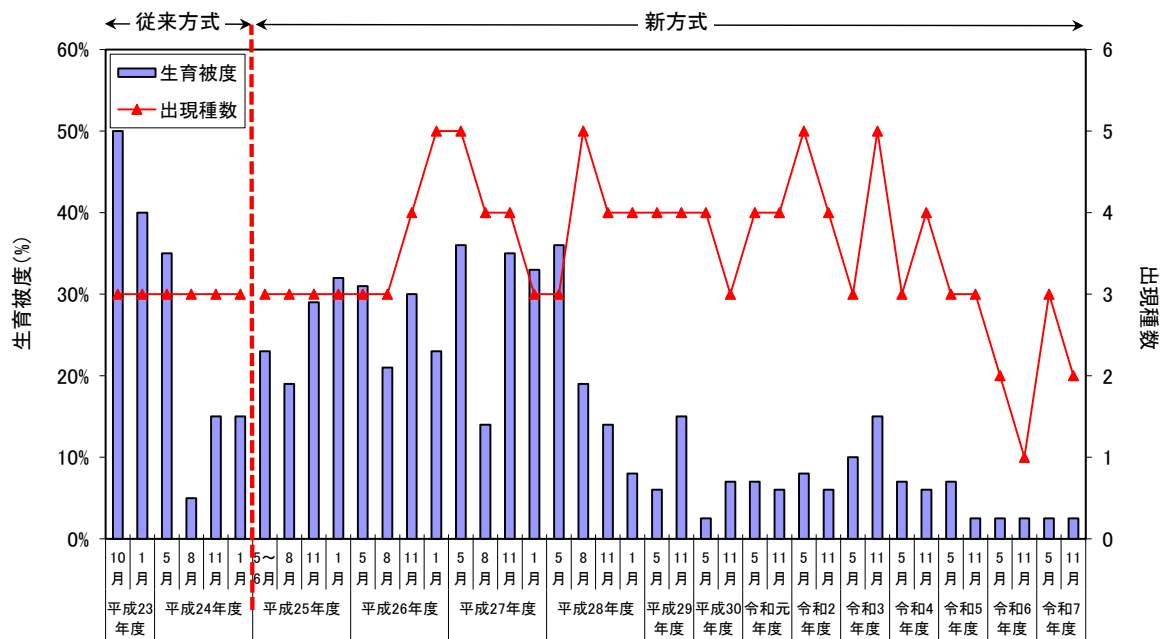
図 2.5.14 小型海草藻場の生育被度の経年変化
