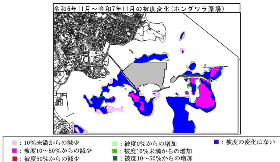
図 2.5.8(2) ホンダワラ藻場の被度変化（令和 6 年 11 月～令和 7 年 11 月）
