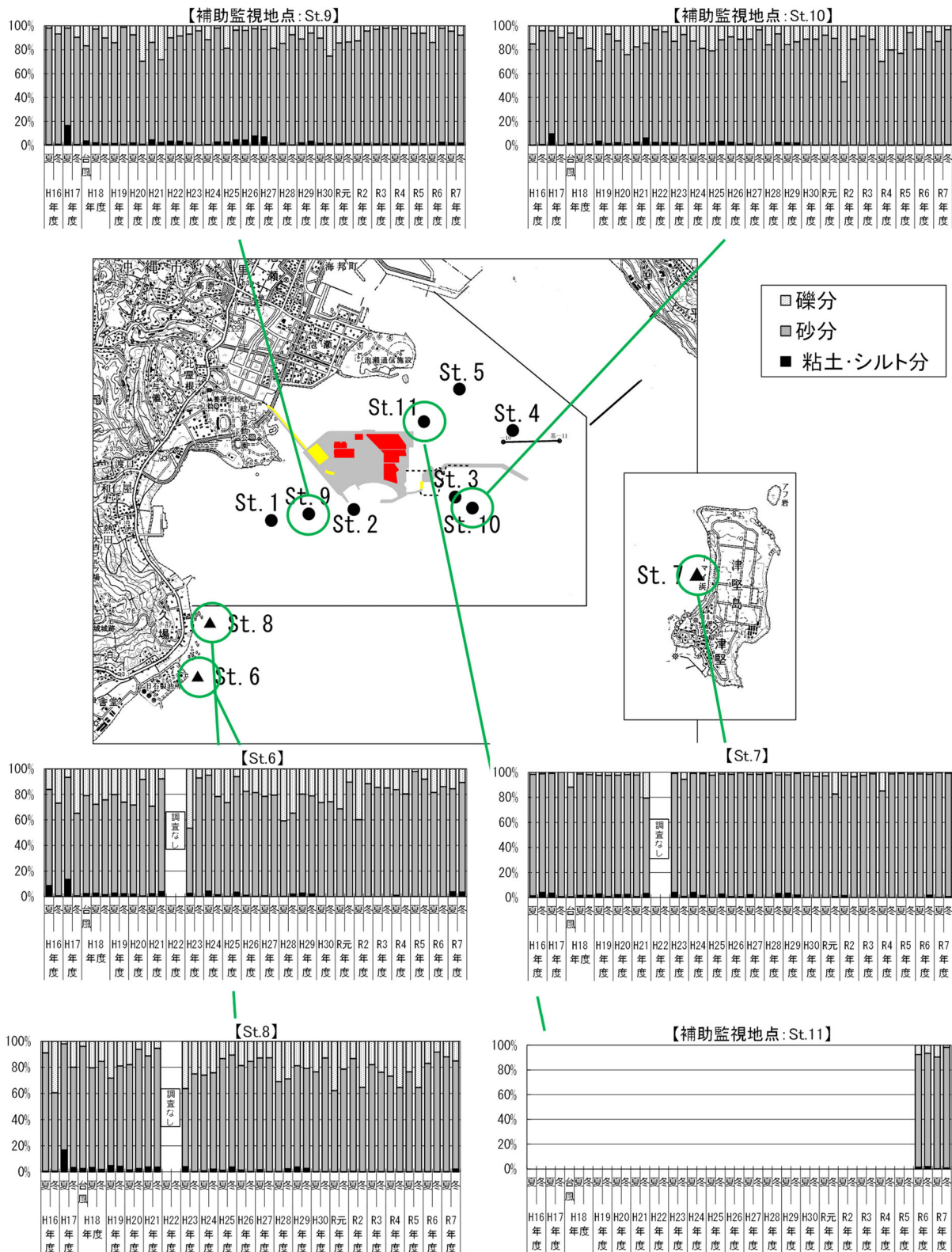
図 2.5.12 (2) 底質の粒度組成調査結果 (St. 6～11)
