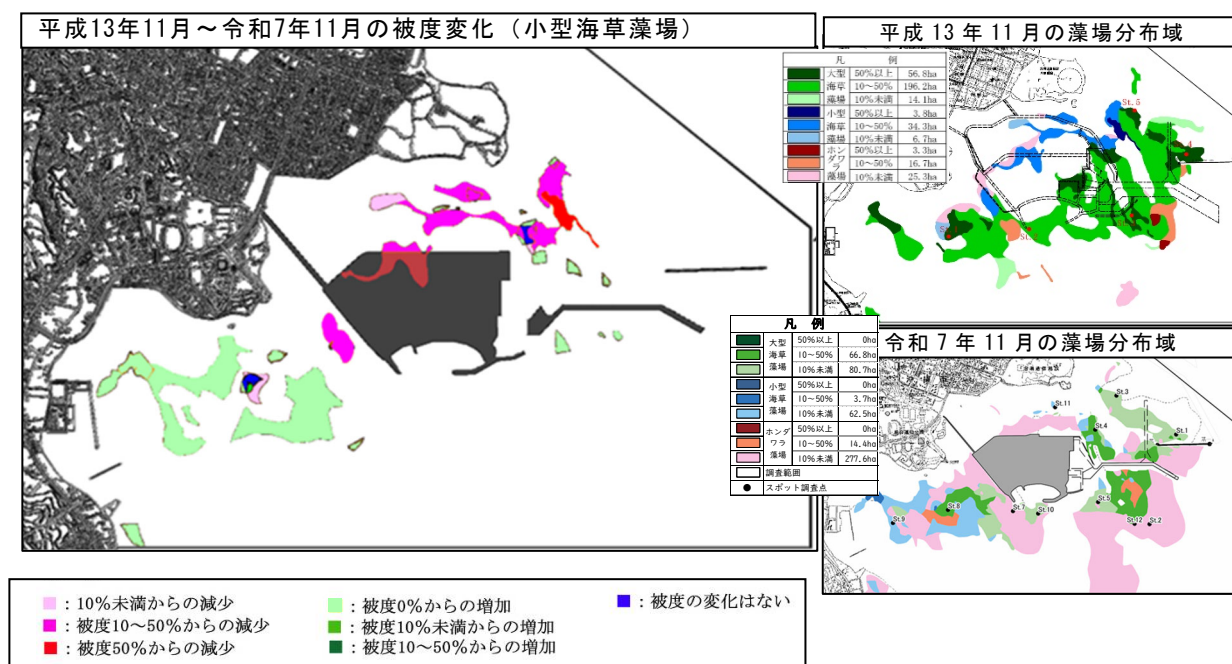
図 2.5.6(1) 小型海草の被度変化（平成13年11月～令和7年11月）
