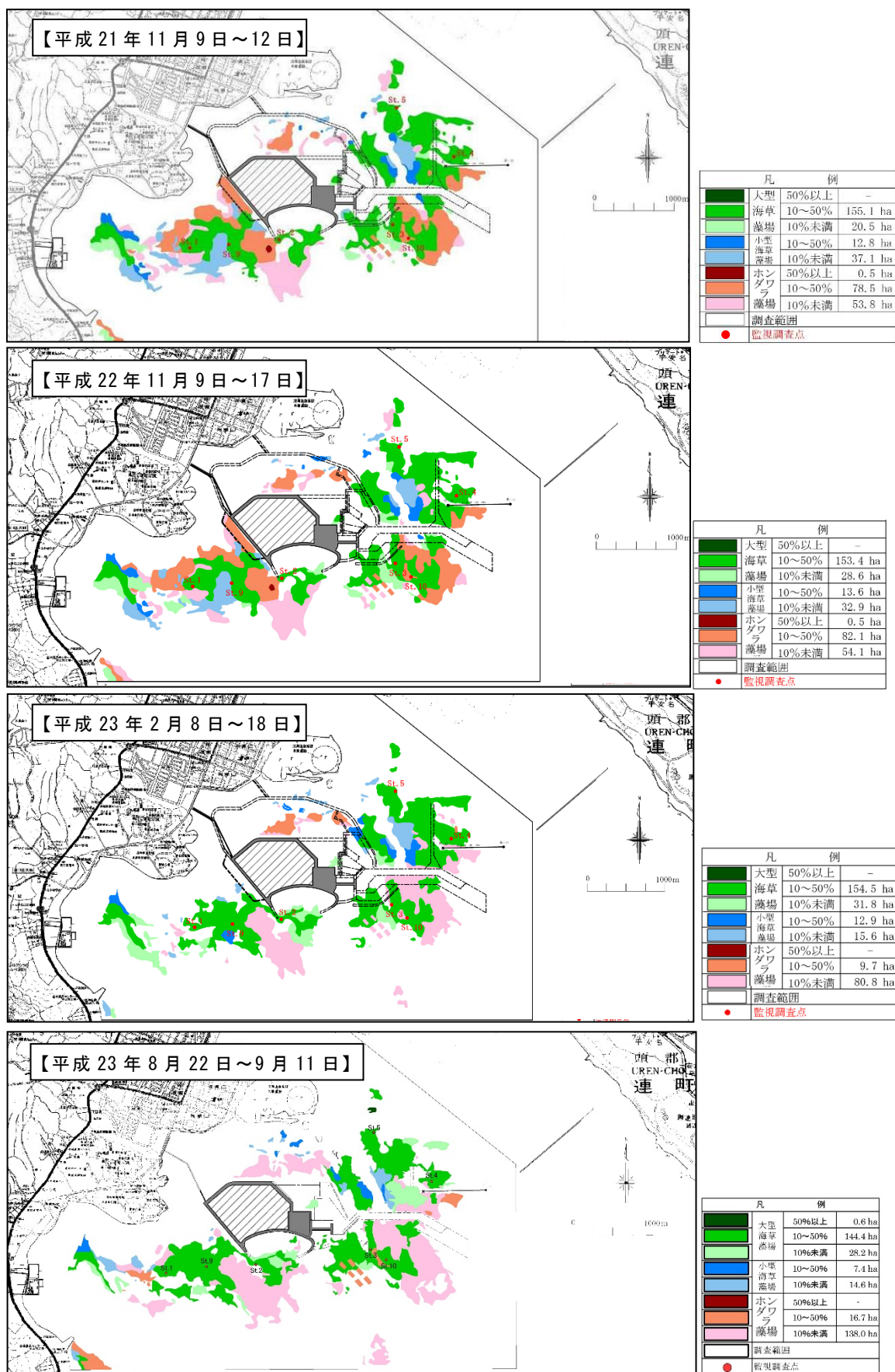
図 2.5.10(5) 海藻草類監視地点（監視区）と藻場分布域
