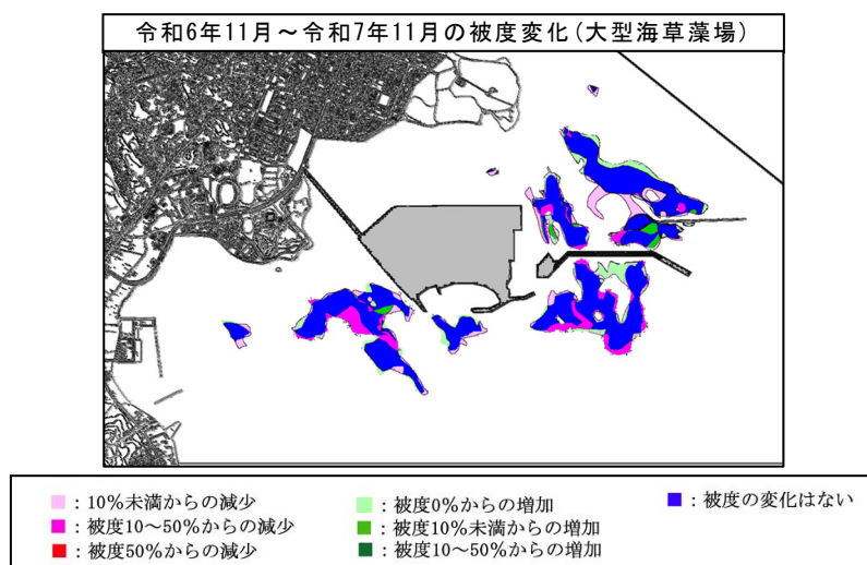
図 2.5.4(2) 大型海草藻場の被度変化（令和 6 年 11 月～令和 7 年 11 月）
