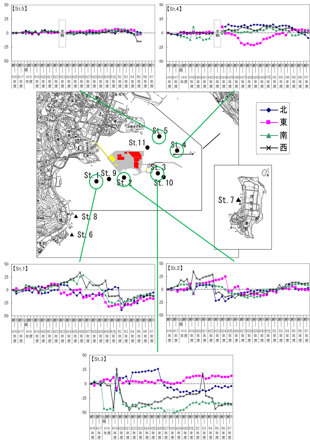
図 2.5.11 (1) 砂面変動の調査結果 (St. 1～5)
