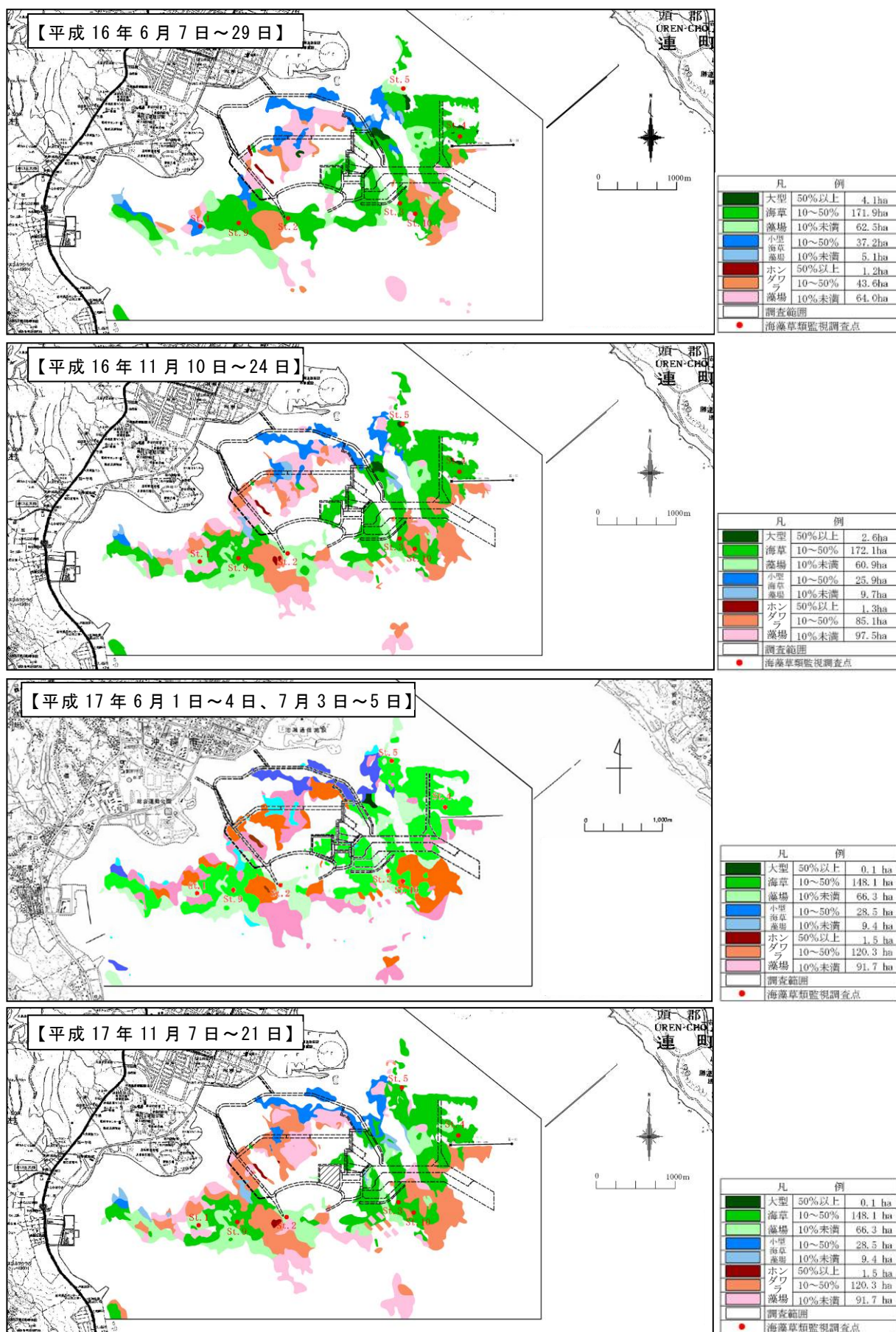
図 2.5.10(2) 海藻草類監視地点（監視区）と藻場分布域
