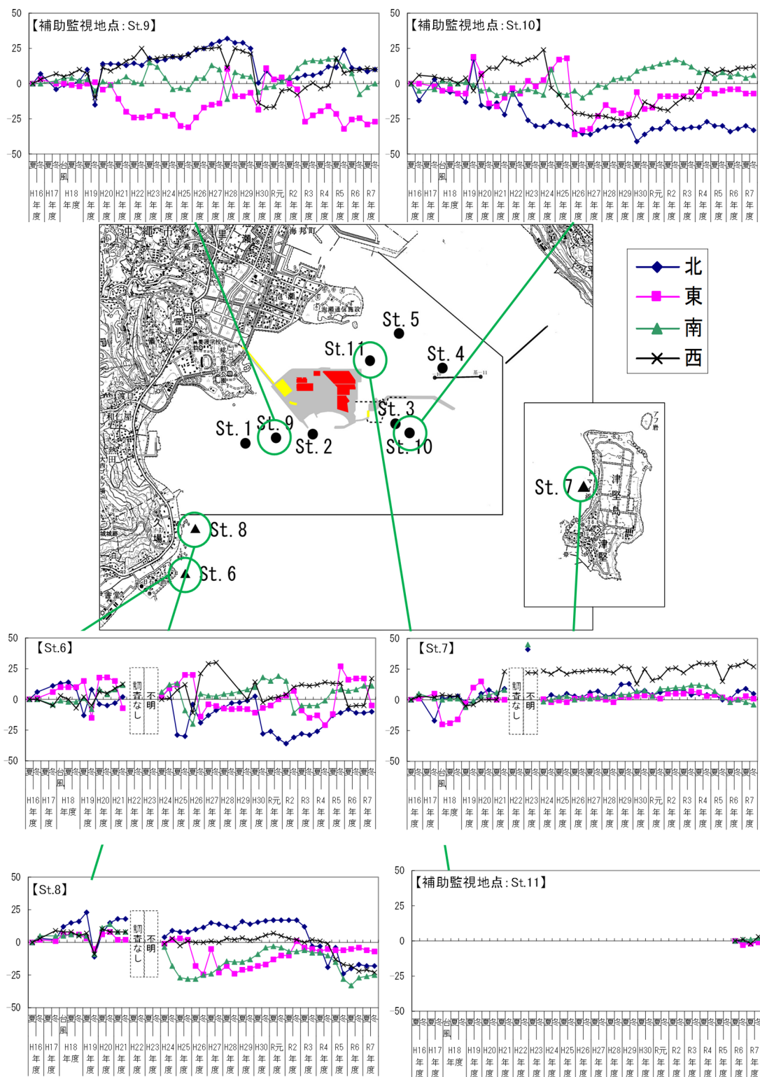
図 2.5.11 (2) 砂面変動の調査結果 (St. 6～11)
