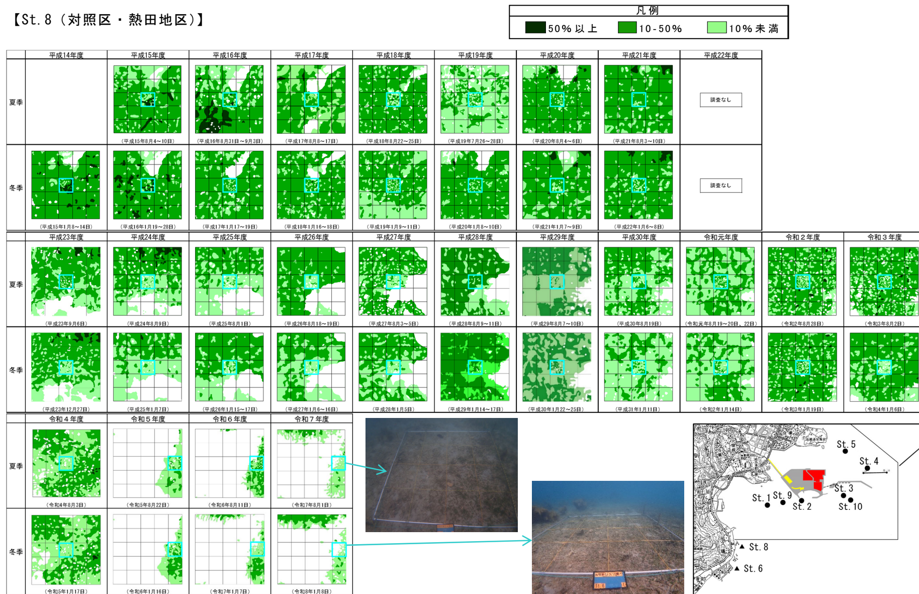
図 2.5.2(8) 各調査地点における過年度からの被度変化の状況
