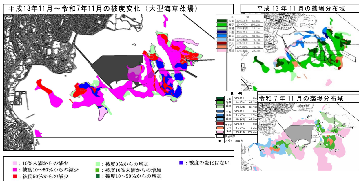
図 2.5.4(1) 大型海草藻場の被度変化（平成 13 年 11 月～令和 7 年 11 月）
