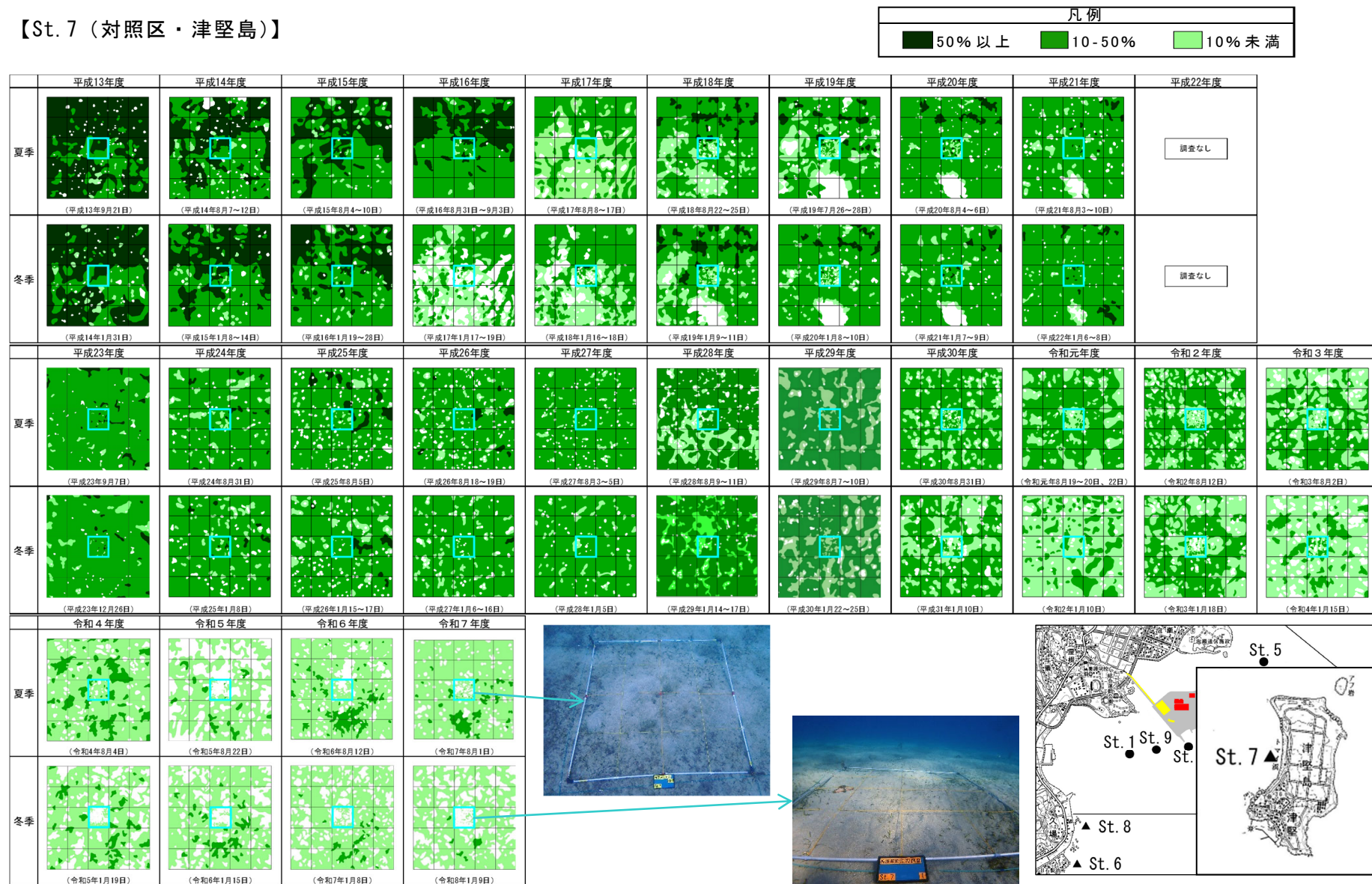
図 2.5.2(7) 各調査地点における過年度からの被度変化の状況
