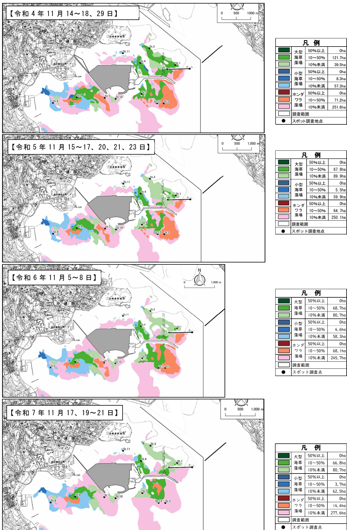
図 2.5.10(10) 海藻草類監視地点（監視区）と藻場分布域
