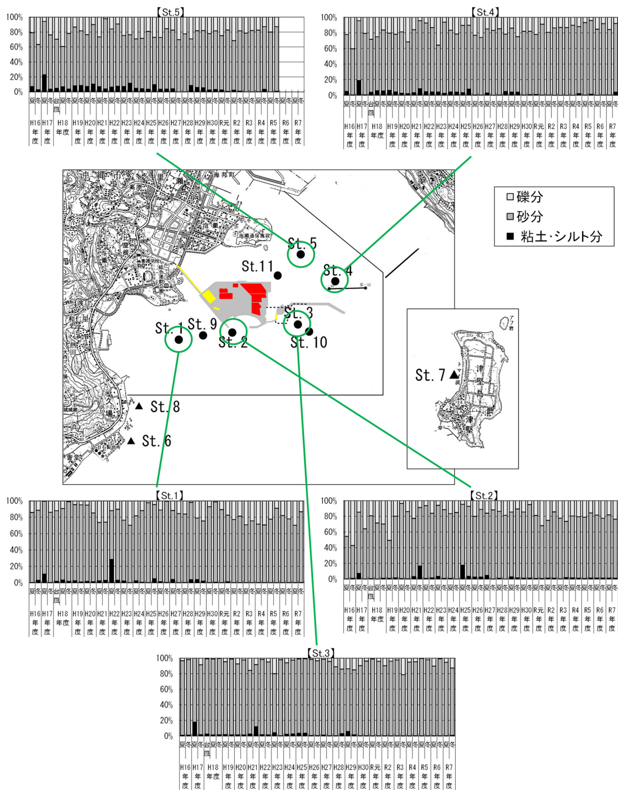
図 2.5.12 (1) 底質の粒度組成調査結果 (St.1～5)
