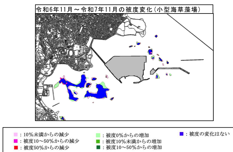
図 2.5.6(2) 小型海草藻場の被度変化（令和6年11月～令和7年11月）
