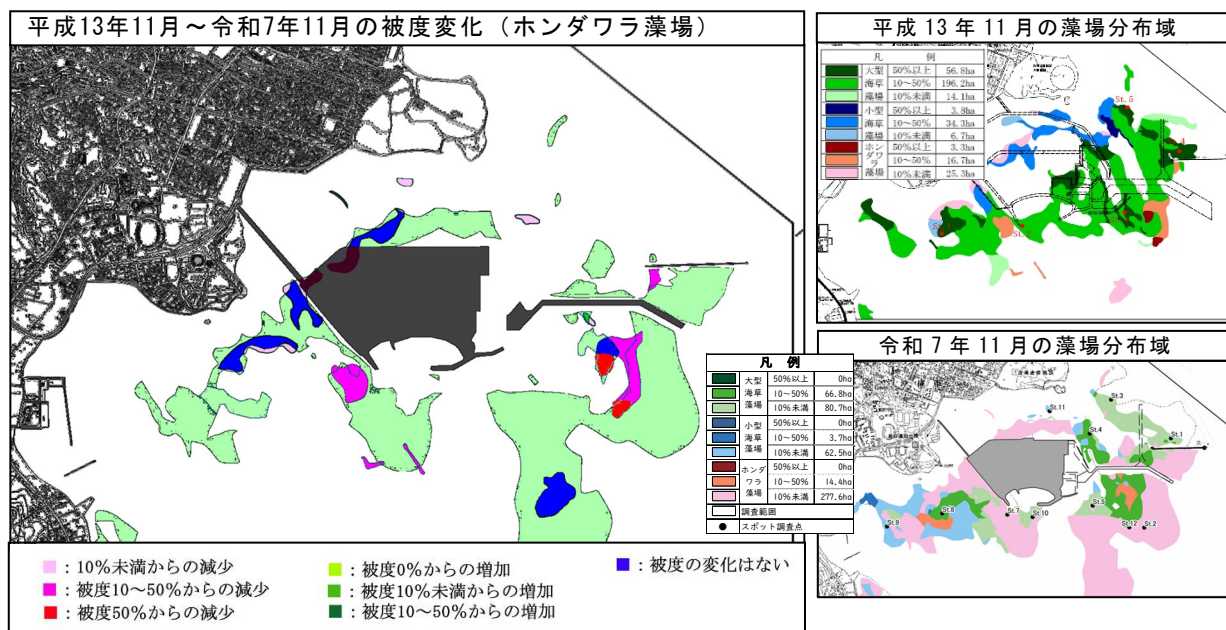
図 2.5.8(1) ホンダワラ藻場の被度変化（平成 13 年 11 月～令和 7 年 11 月）
