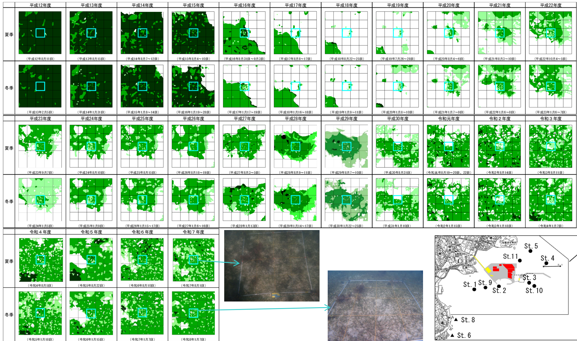
図 2.5.2(3) 各調査地点における過年度からの被度変化の状況
