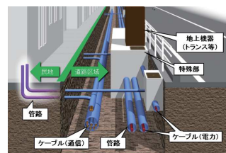
電線共同溝（イメージ）
