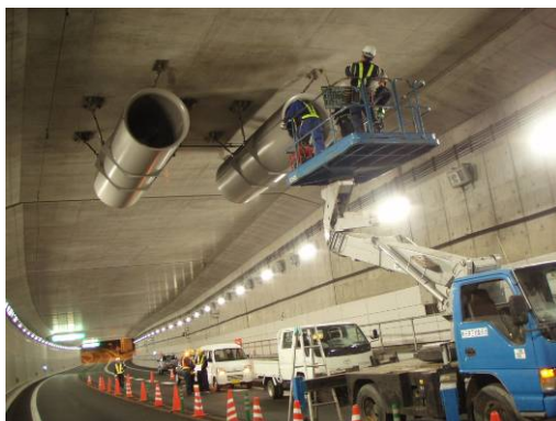
【トンネル非常用施設 (換気設備) 点検】
