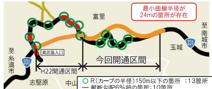
▲ 中山改良並行区間における線形不良箇所
