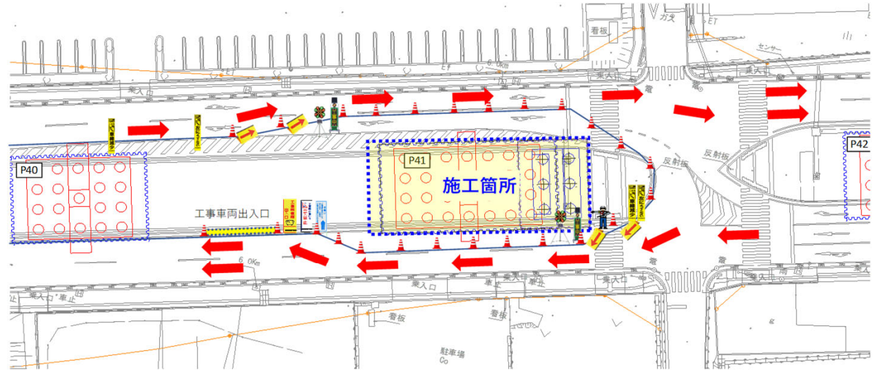
交通規制図
