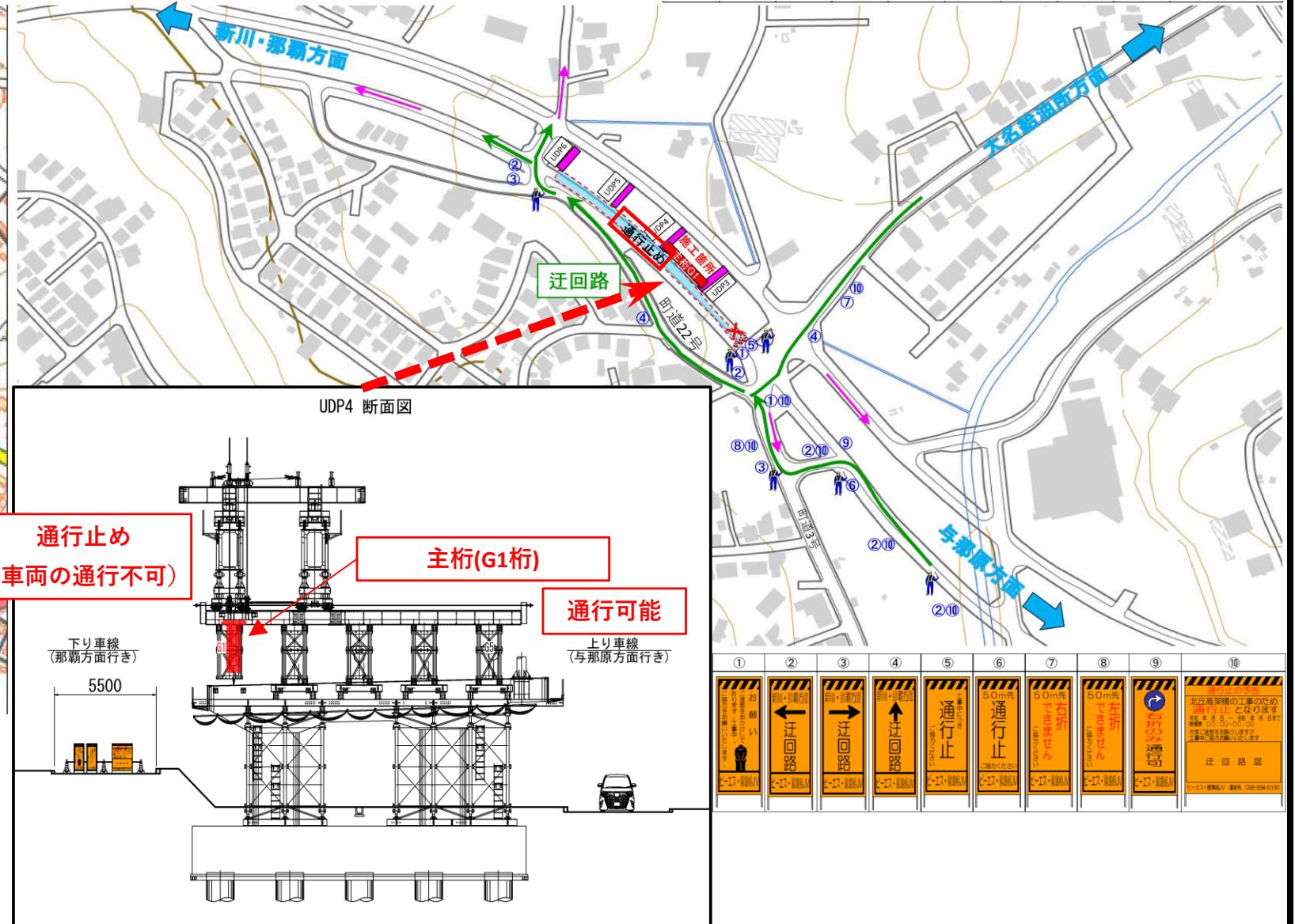
交通規制図
