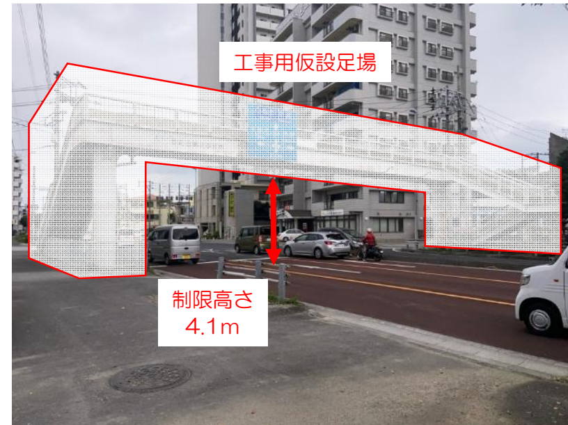
交通規制（高さ制限）概要図
