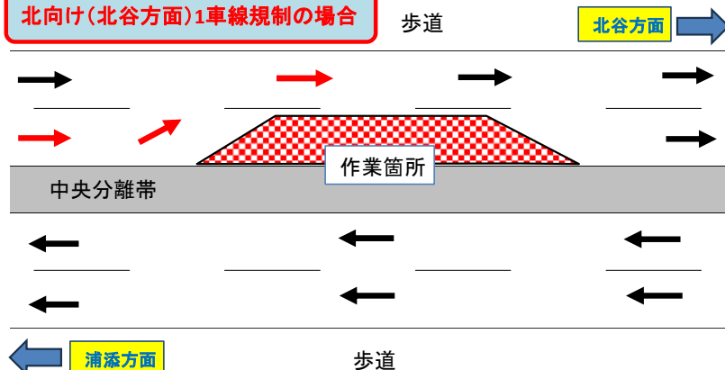
交通規制概要図
