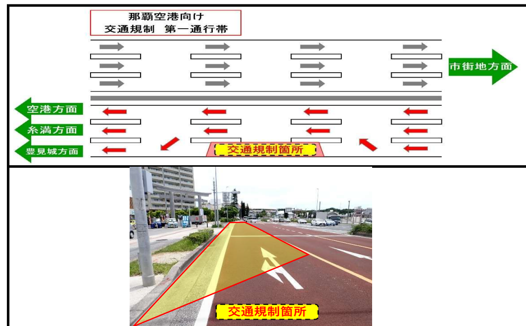
交通規制図
