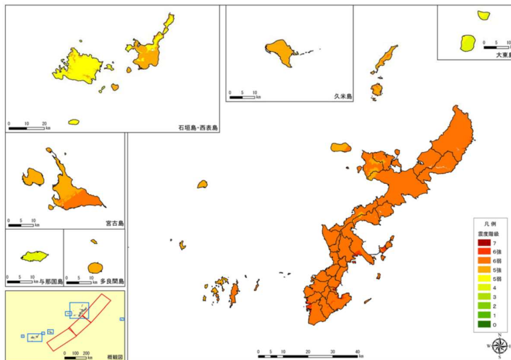
図3 沖縄本島南東沖地震3連動の震度分布図
