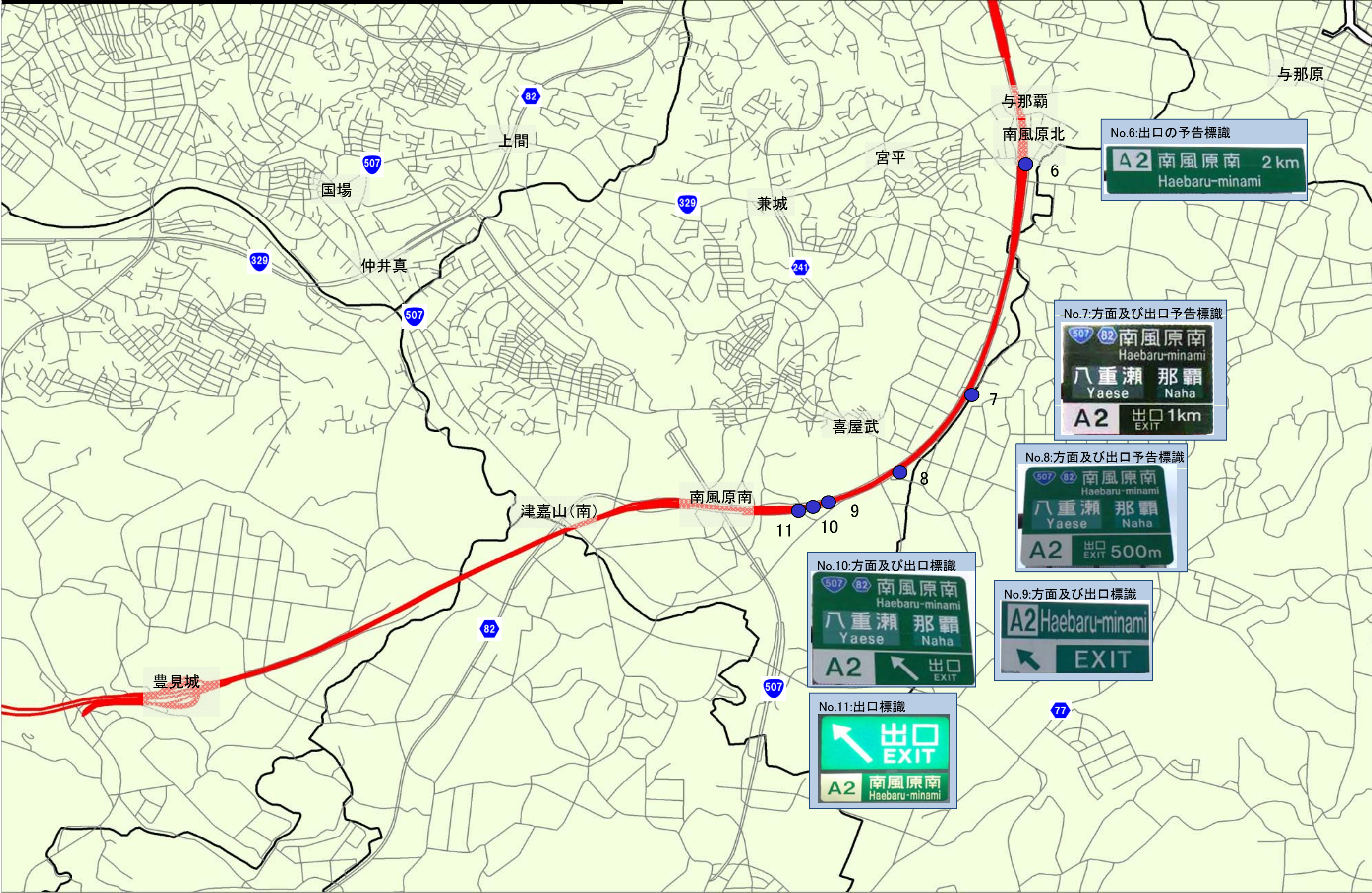
国道506号(上り)道路案内標識現況位置図(2／3)
