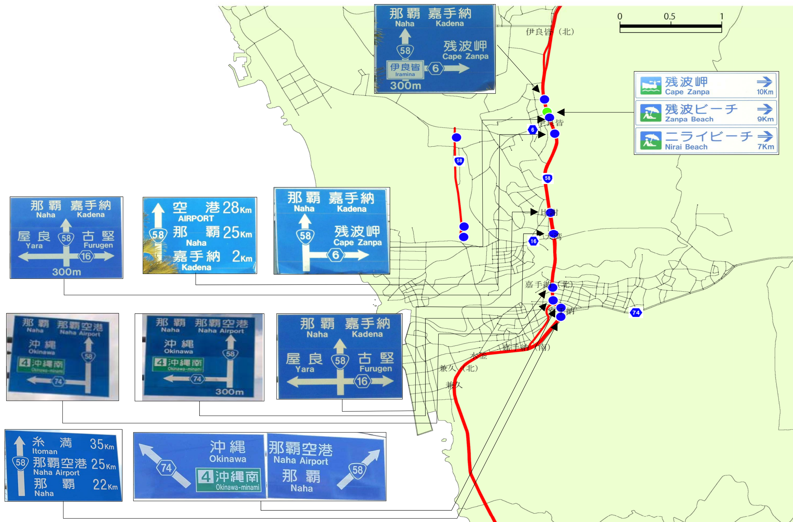
国道58号(下り)道路案内標識現況位置図(13/21)
